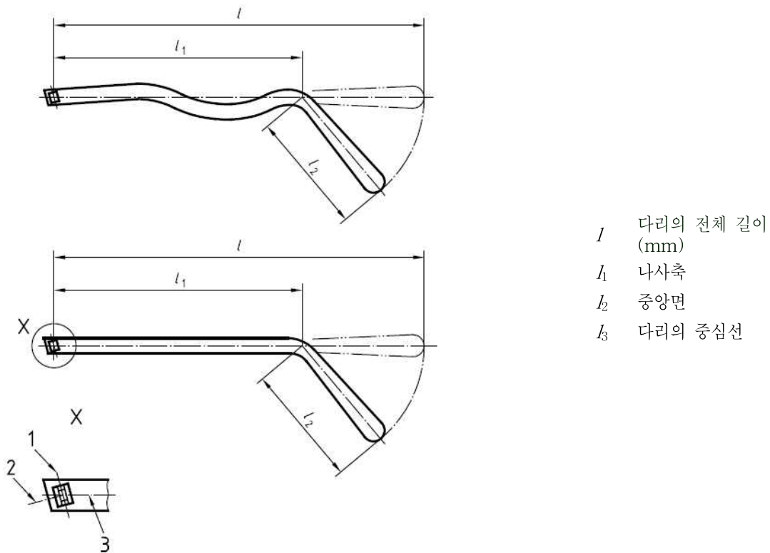
그림 2 안경테 치수의 측정 (다리)
